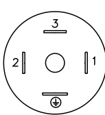
E – EN 175301-803 Tipo A M – EN 175301-803 Tipo C-ind
